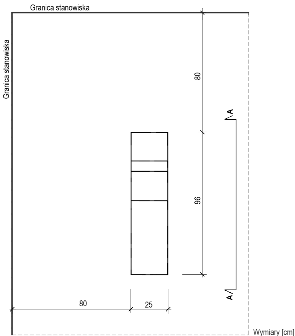
Rysunek 1. Usytuowanie muru na stanowisku egzaminacyjnym (rzut)
