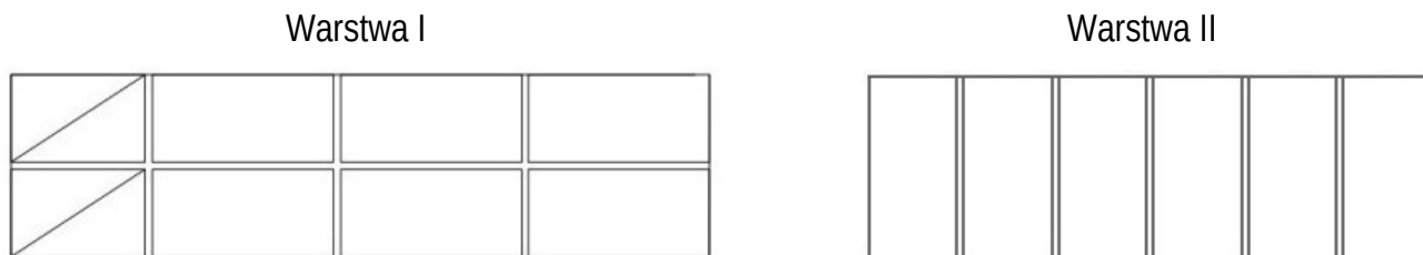
Rysunek 2. Układ cegieł w pierwszej i drugiej warstwie muru (rzuty)
