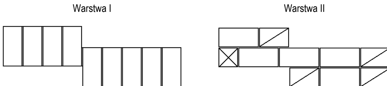
Rysunek 2. Układ cegieł w pierwszej i drugiej warstwie muru (rzuty)
