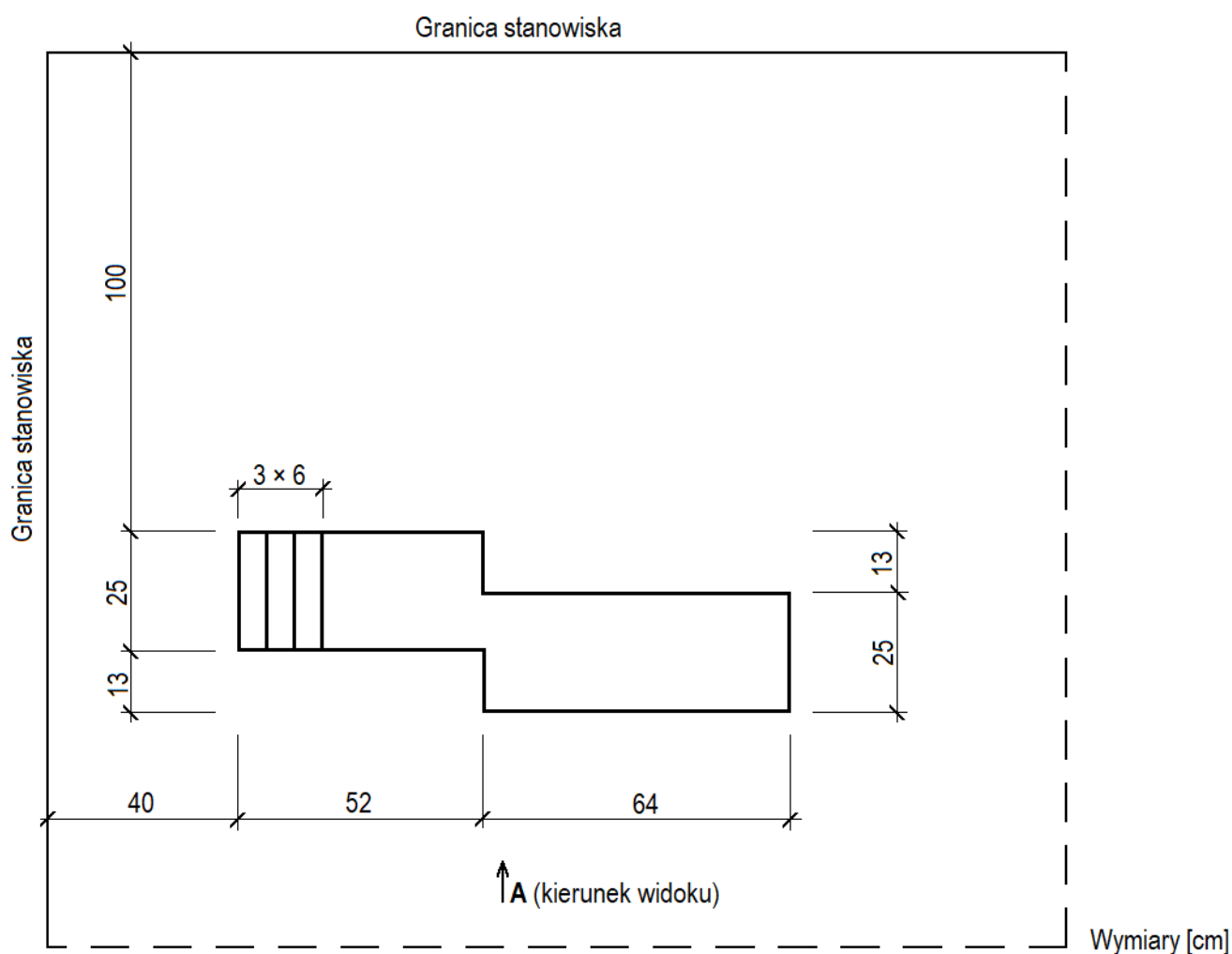
Rysunek 1. Usytuowanie muru na stanowisku egzaminacyjnym (rzut)
