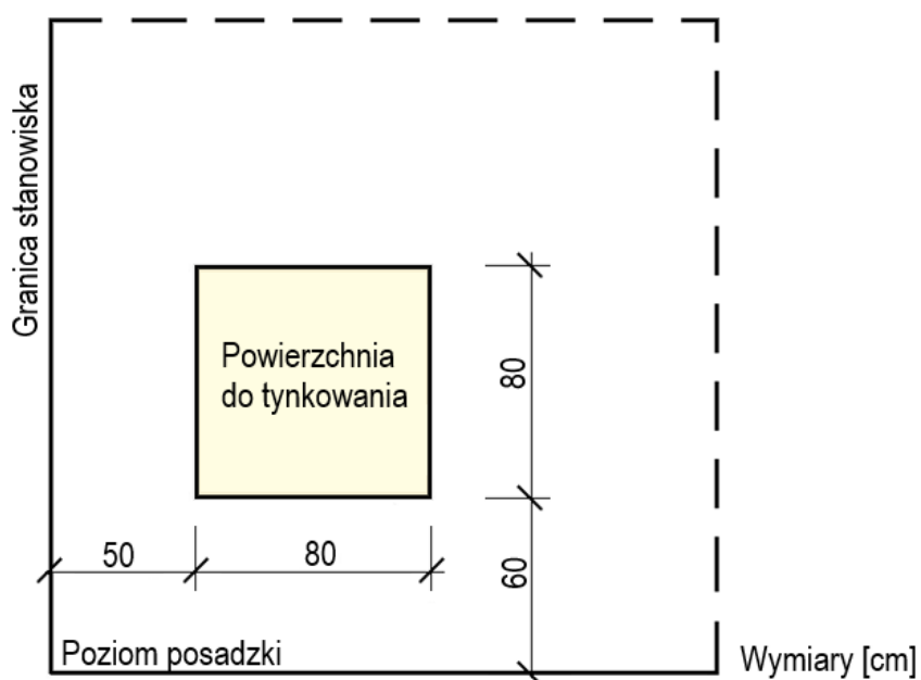
Rysunek 4. Usytuowanie powierzchni tynku na ścianie (widok)
