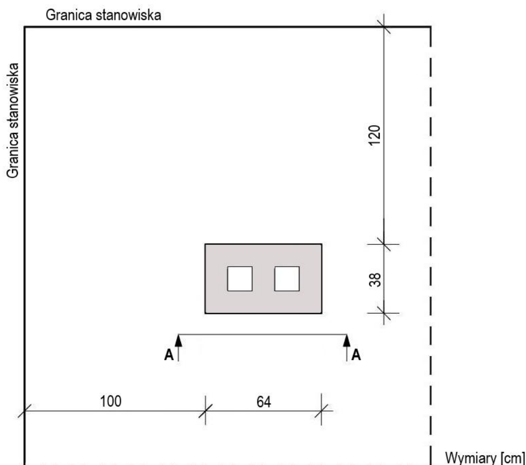
Rysunek 1. Usytuowanie komina na stanowisku egzaminacyjnym (rzut)
