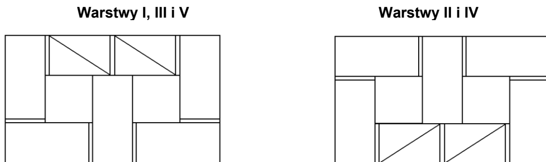
Rysunek 2. Układ cegieł w kolejnych warstwach komina (rzuty)
