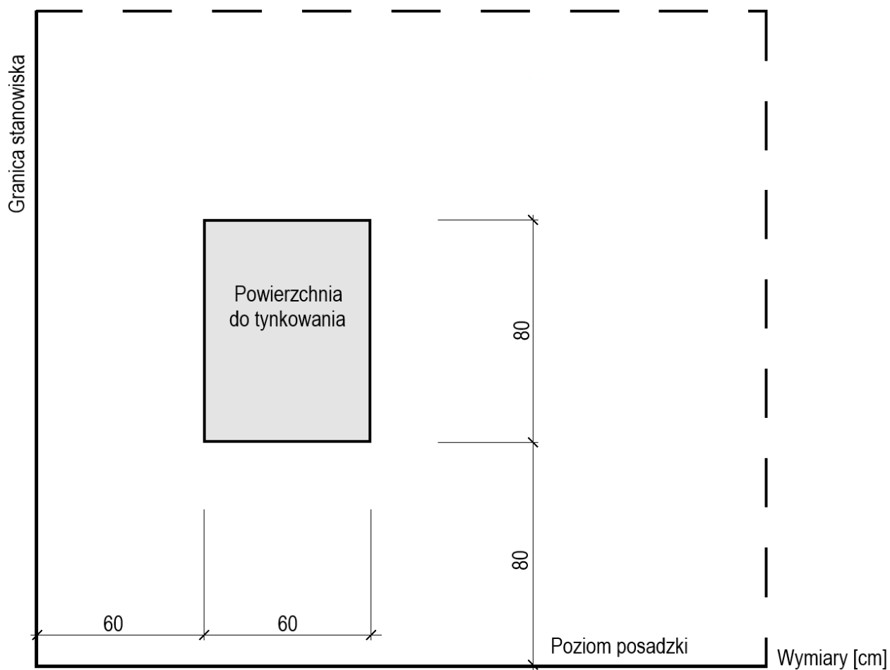
Rysunek 4. Usytuowanie powierzchni tynku na ścianie (widok)
