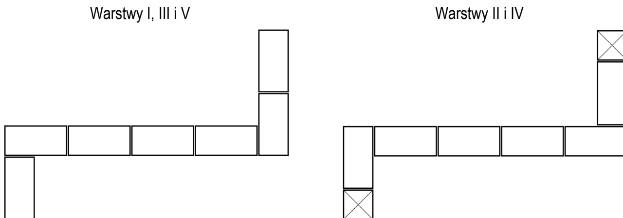
Rysunek 2. Układ cegieł w kolejnych warstwach ścianki działowej (rzuty)
