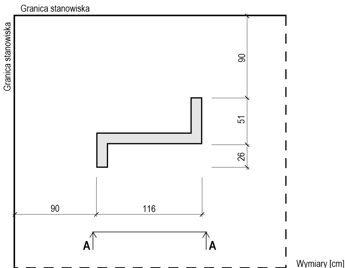
Rysunek 1. Usytuowanie ścianki działowej na stanowisku egzaminacyjnym (rzut)
