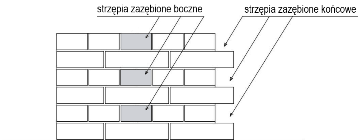
Rysunek 3. Widok A-A lica muru
