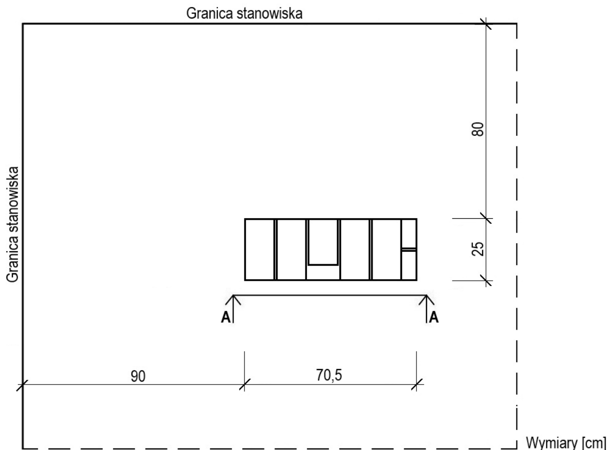
Rysunek 1. Usytuowanie muru na stanowisku egzaminacyjnym (rzut)
