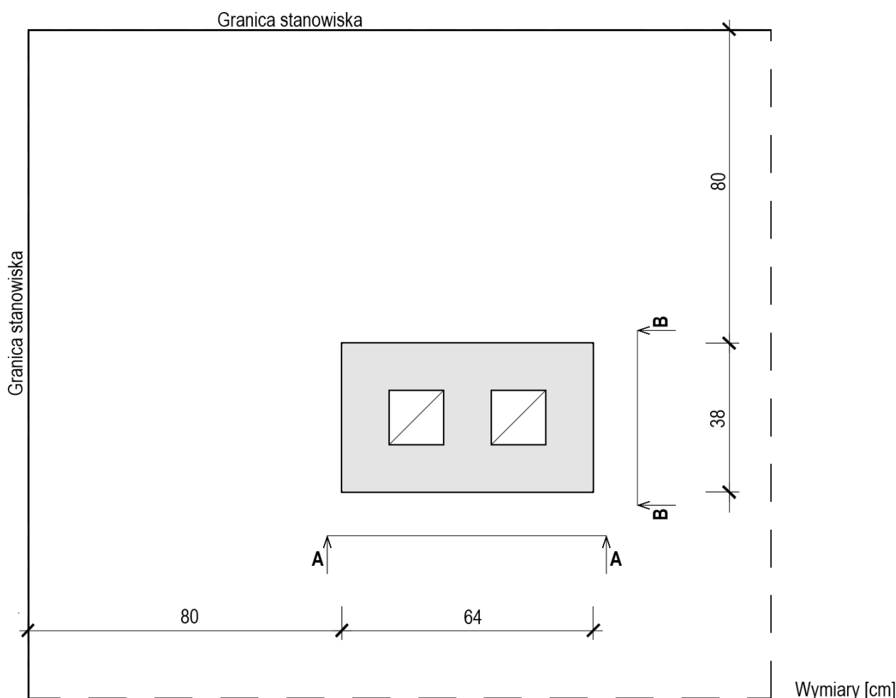
Rysunek 1. Usytuowanie komina na stanowisku egzaminacyjnym (rzut)
