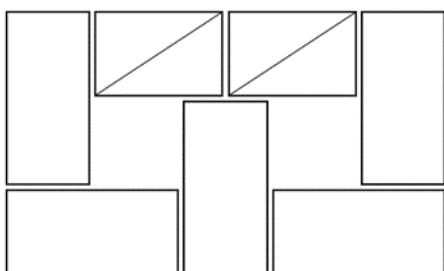
Rysunek 2. Układ cegieł w kolejnych warstwach komina (rzuty)
