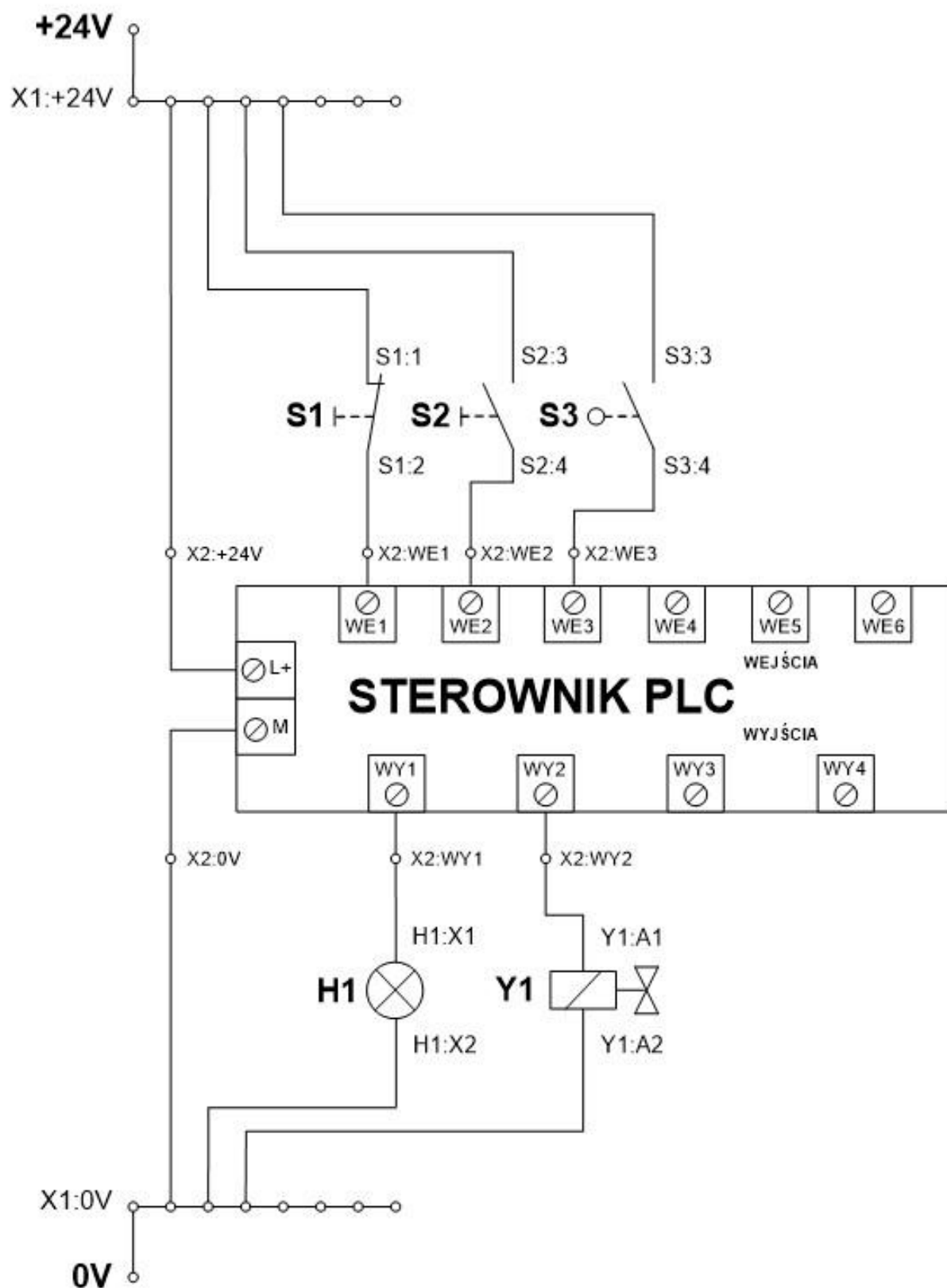
Rysunek 2. Schemat elektryczny układu sterowania automatyki przemysłowej
