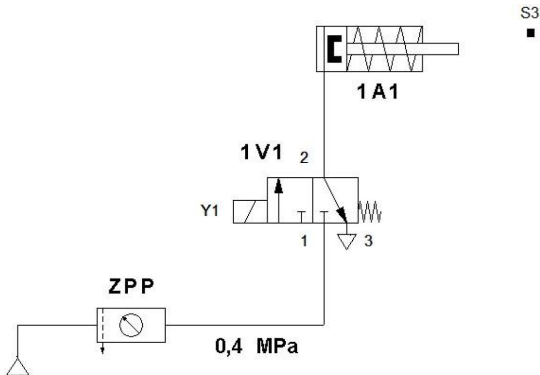
Rysunek 3. Schemat pneumatyczny układu sterowania automatyki przemysłowej
