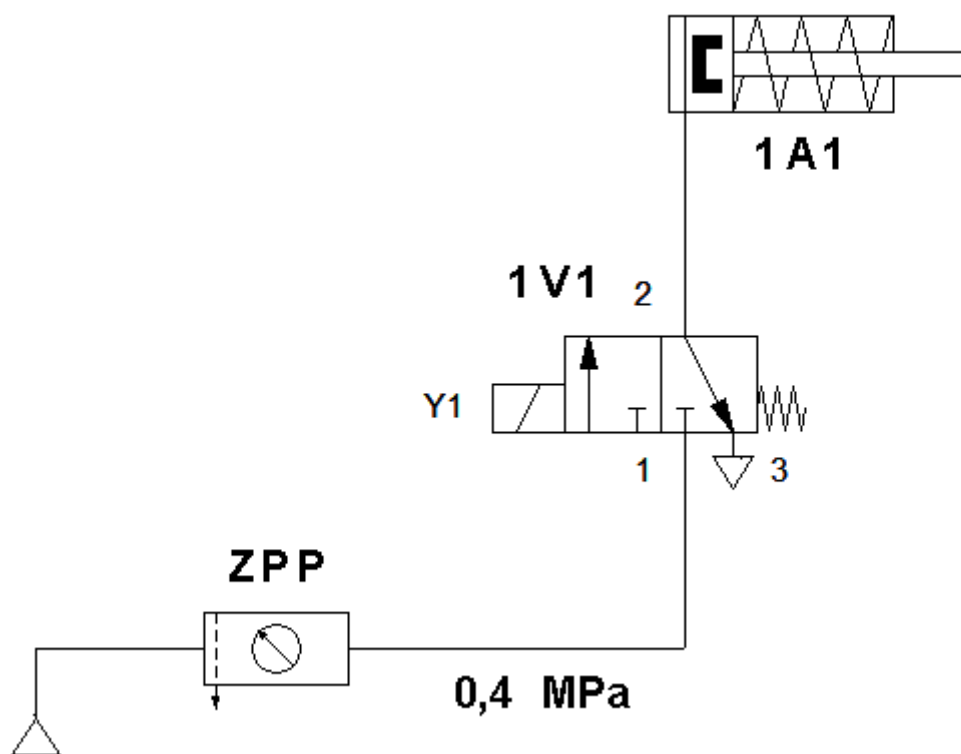
Rysunek 3. Schemat pneumatyczny układu sterowania automatyki przemysłowej
