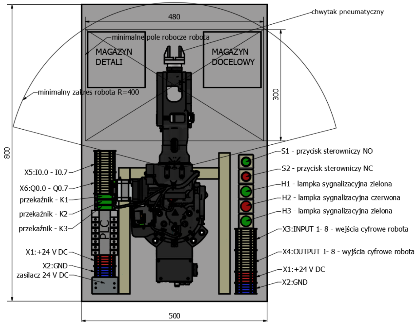
Rysunek 6. Stanowisko zrobotyzowane do układania detali
