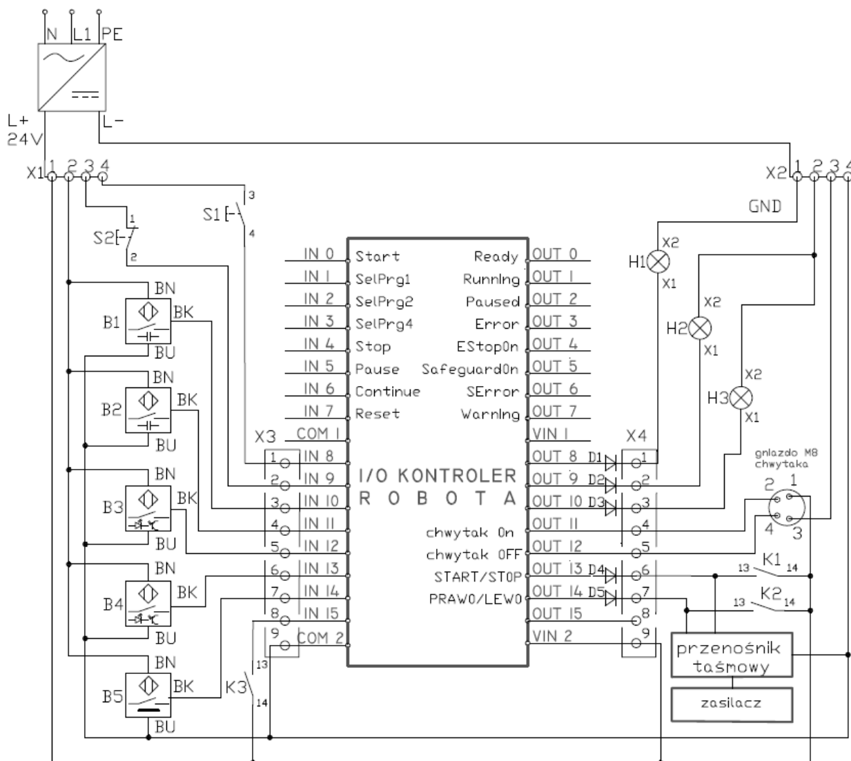
Rysunek 4. Schemat elektryczny systemu zrobotyzowanego
