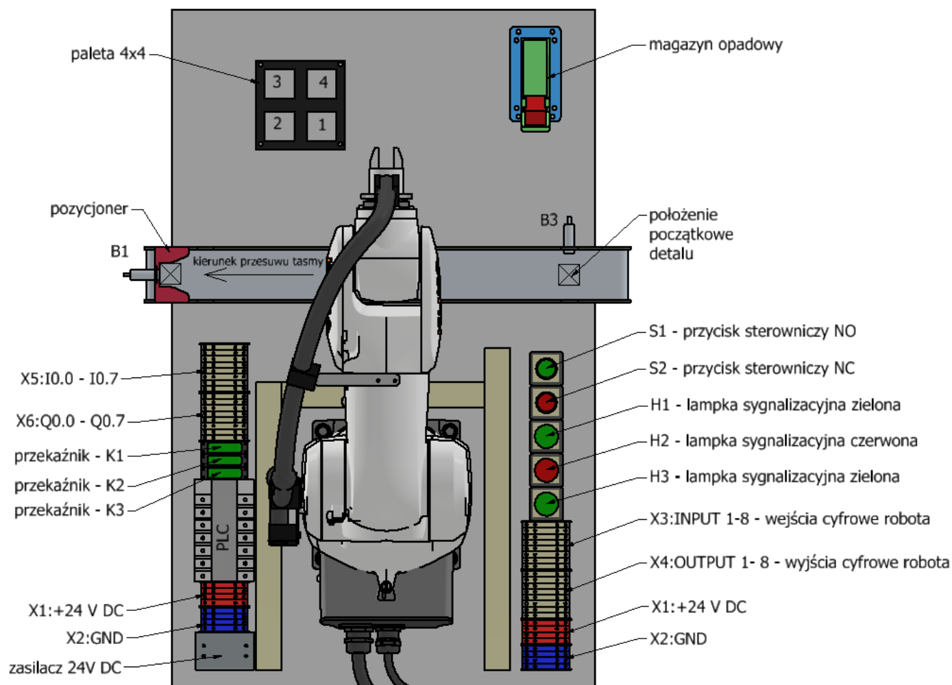
Rysunek 2. Widok płyty z robotem i zamontowanymi elementami systemu zrobotyzowanego
