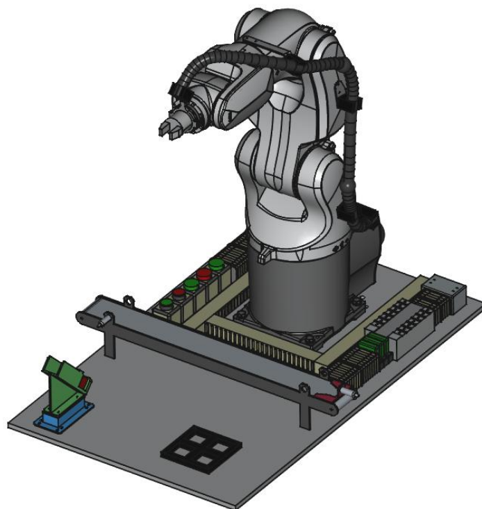
Rysunek 1. Poglądowy widok zrobotyzowanego stanowiska paletyzacji
