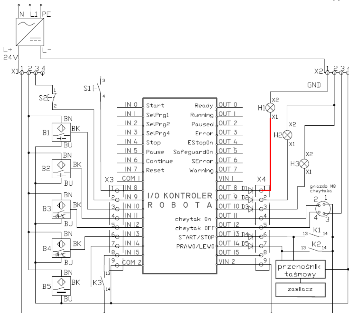
Rysunek 5. Schemat połączeń elektrycznych systemu zrobotyzowanego
