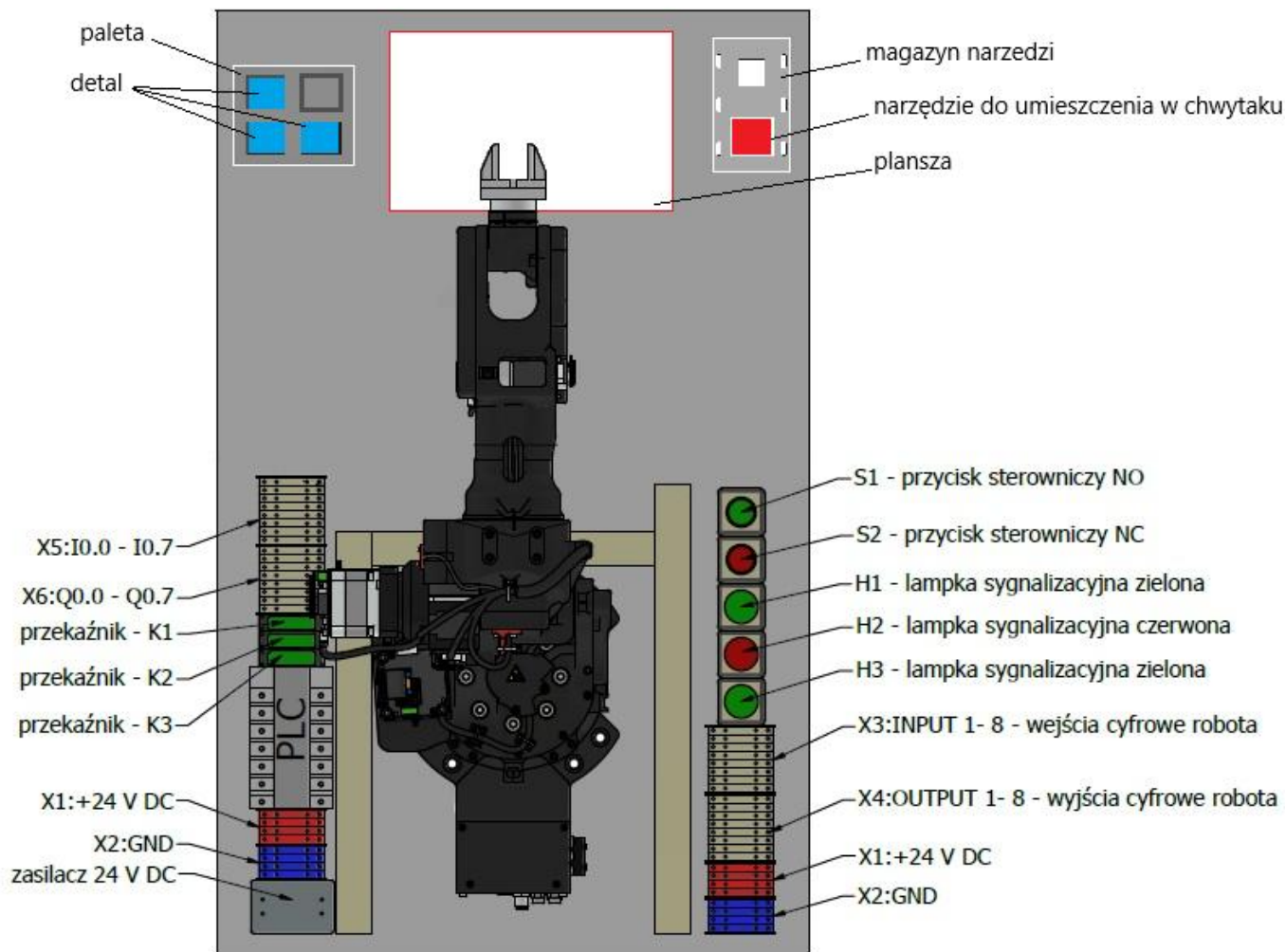
Rysunek 1. Rozmieszczenie komponentów stanowiska
