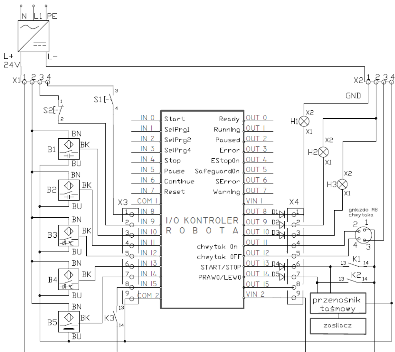
Rysunek 4. Schemat połączeń elektrycznych systemu zrobotyzowanego
