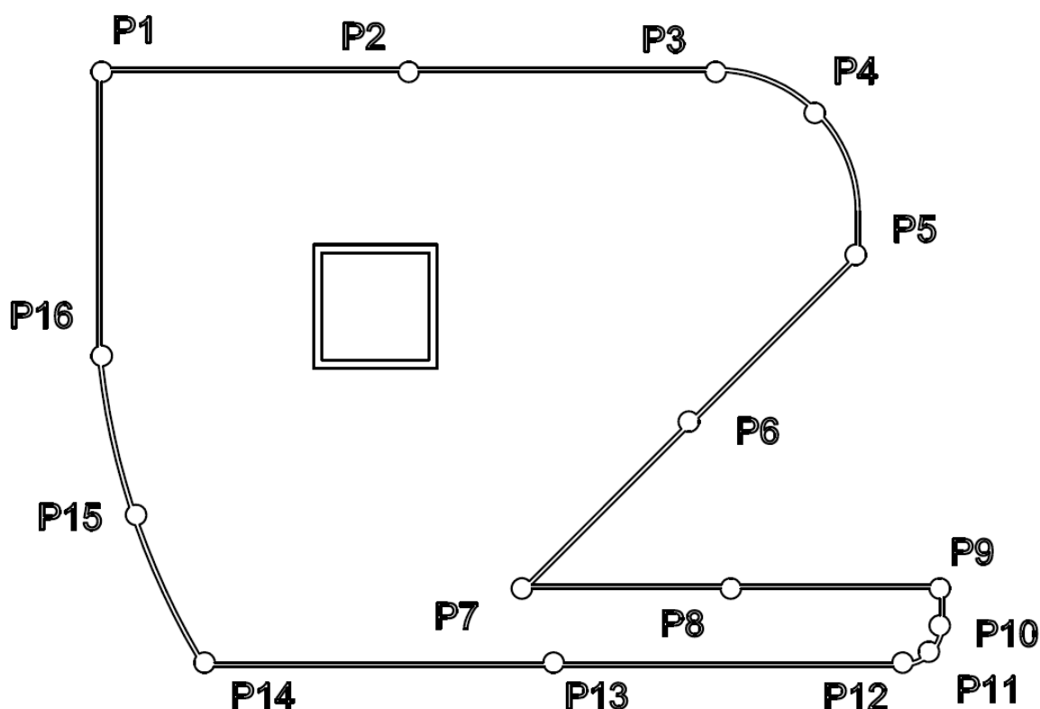
Rysunek 4. Plansza nr 1 z torem ruchu robota.
