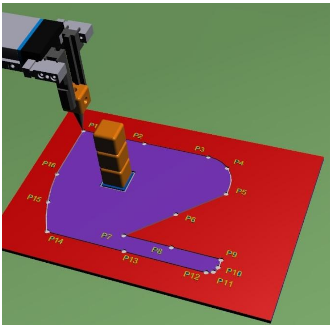
Rysunek 3. Etap drugi zadania – przemieszczanie narzędzia między punktami
