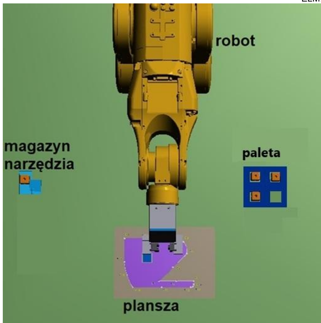
Rysunek 5. Rozmieszczenie elementów stanowiska
