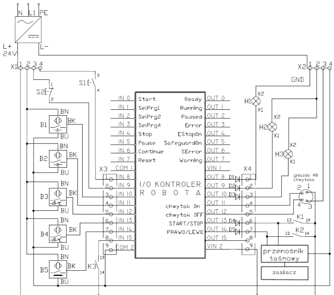
Rysunek 2. Schemat połączeń elektrycznych systemu zrobotyzowanego
