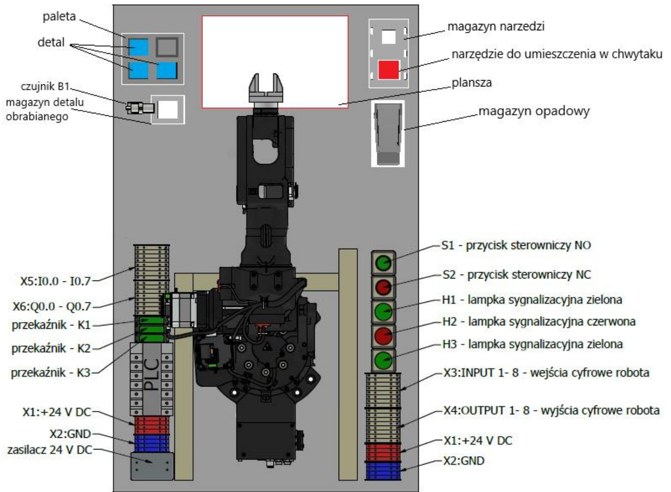
Rysunek 5. Rozmieszczenie elementów stanowiska
