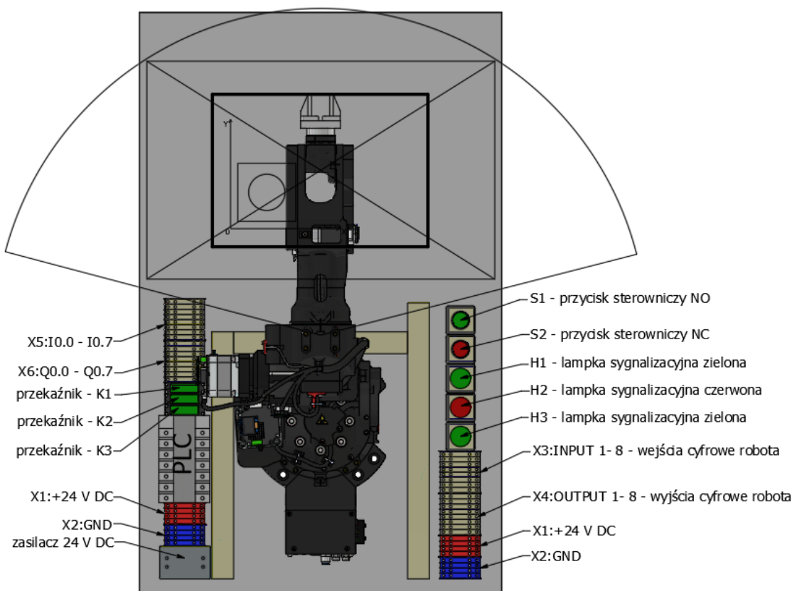
Rysunek 1. Przestrzeń robocza przed robotem
