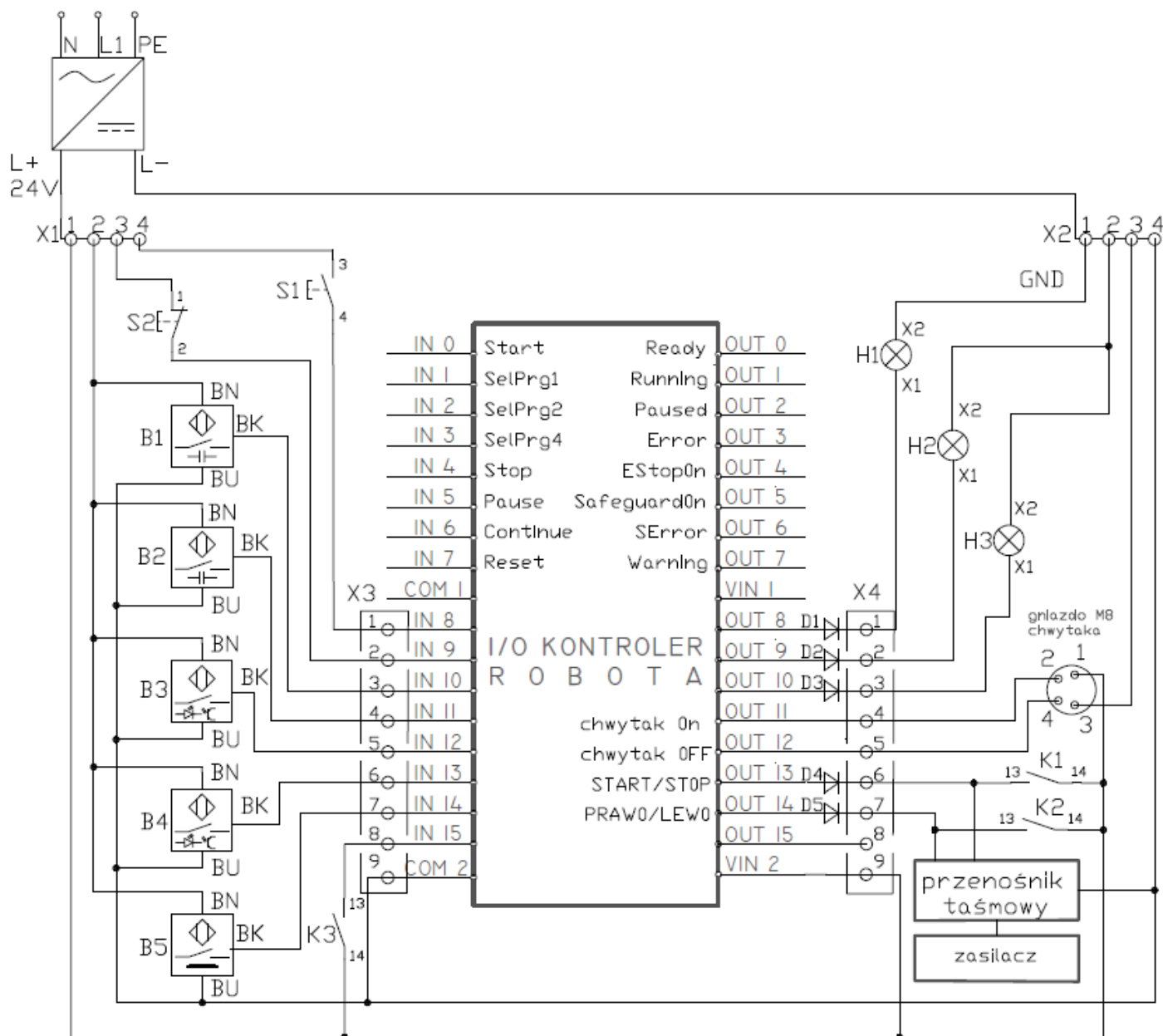
Rysunek 2. Schemat podłączenia kontrolera robota
