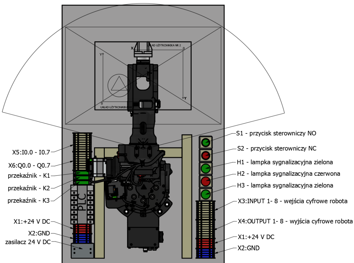
Rysunek 1. Przestrzeń robocza przed robotem
